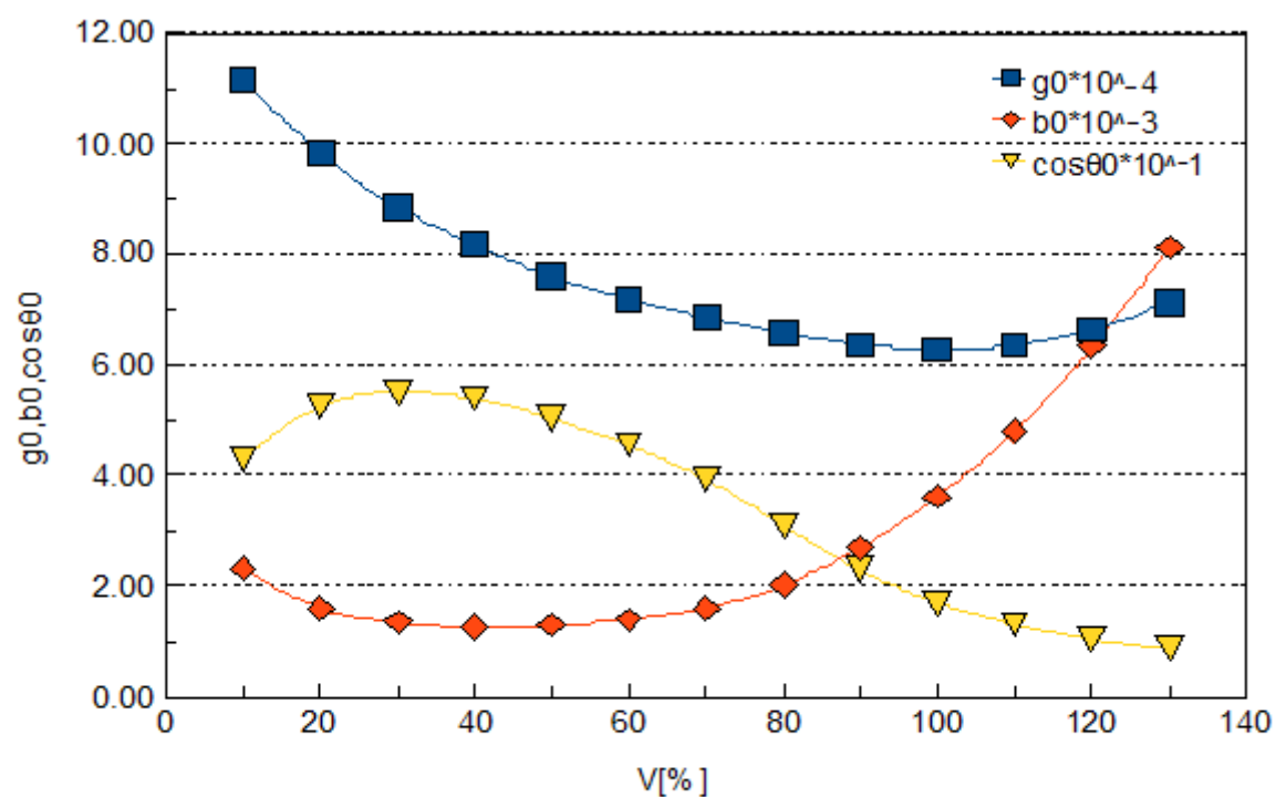
図6.1 解放試験(a)の測定結果
