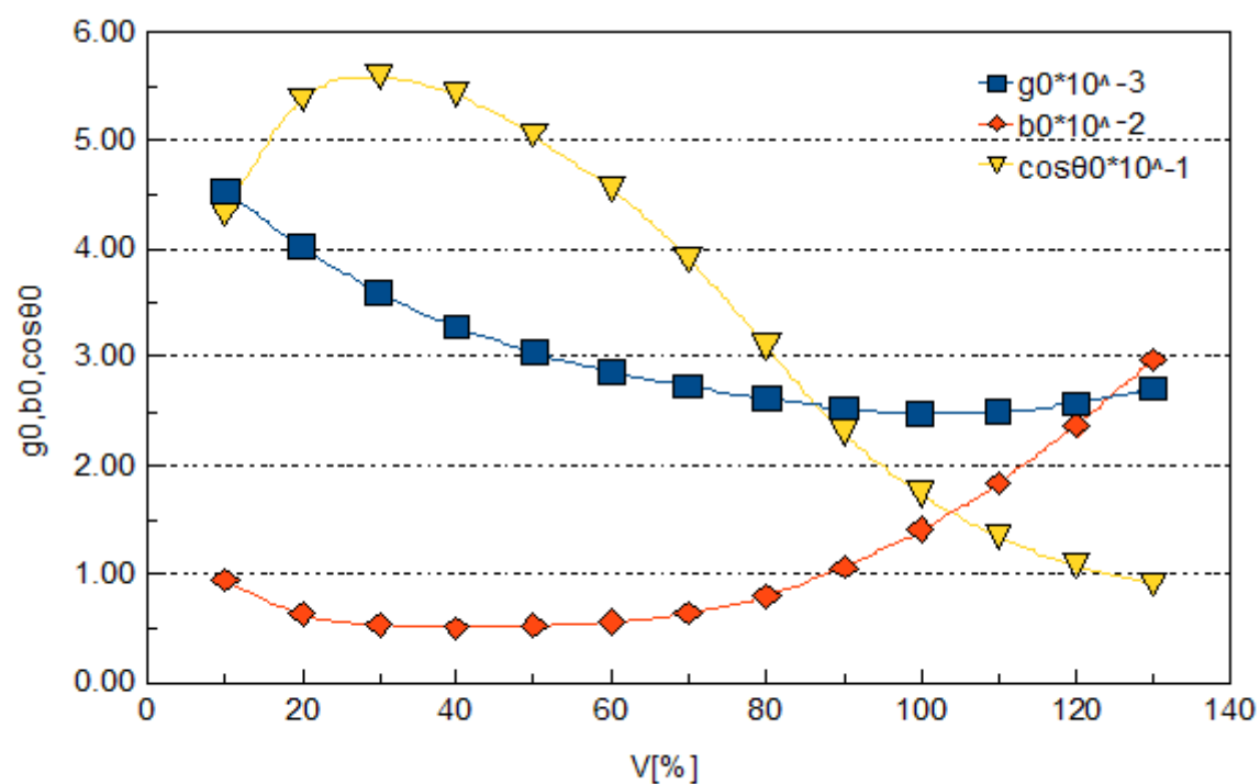
図6.2 解放試験(b)の測定結果
