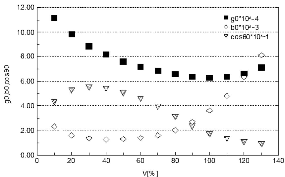
図6.1 開放試験(a)の測定結果
