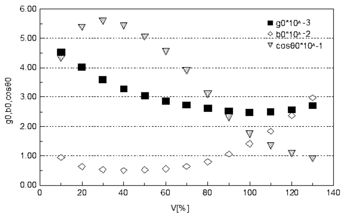
図6.2 開放試験(b)の測定結果
