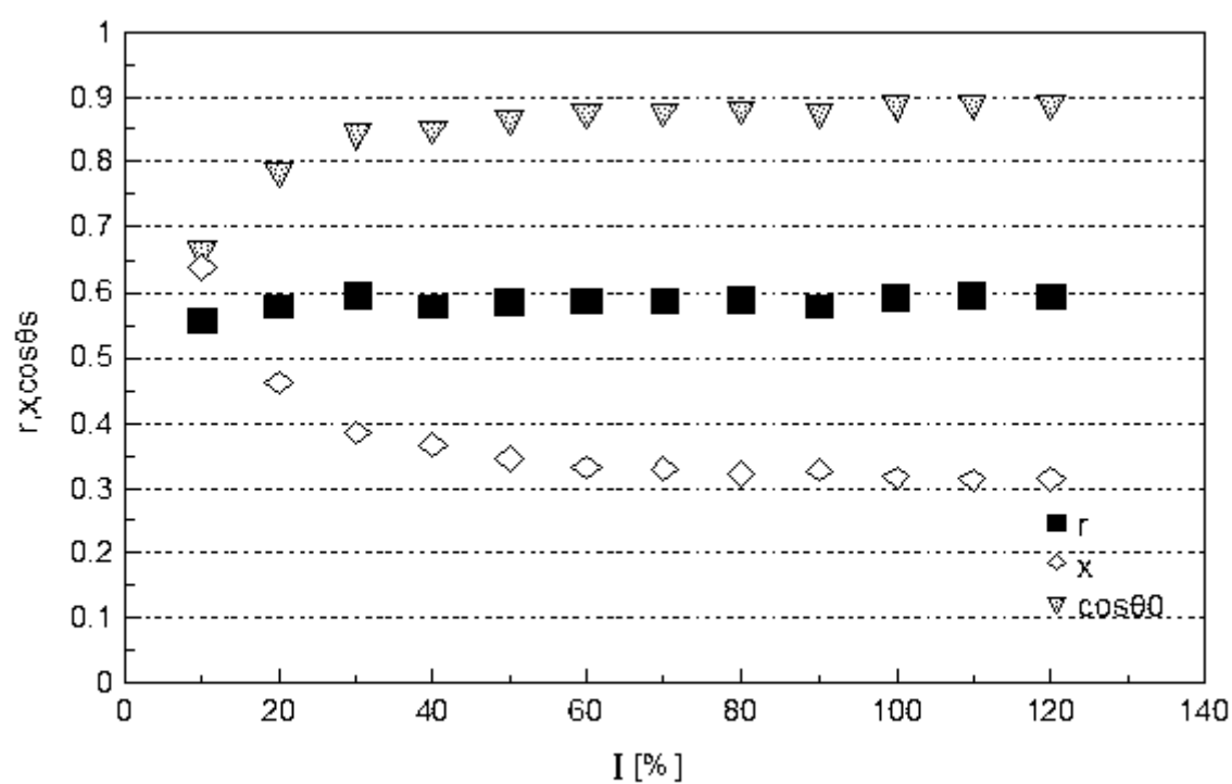
図6.3 短絡試験の測定結果
