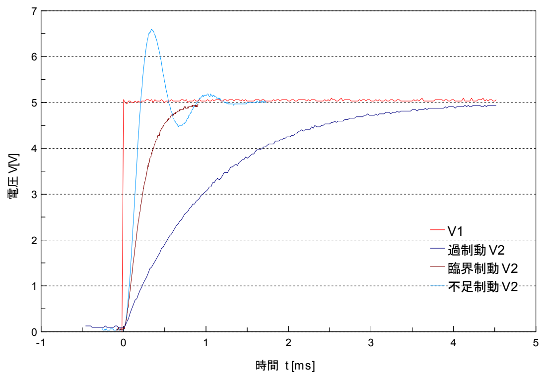
図7. 3 RLCにおける過渡応答
