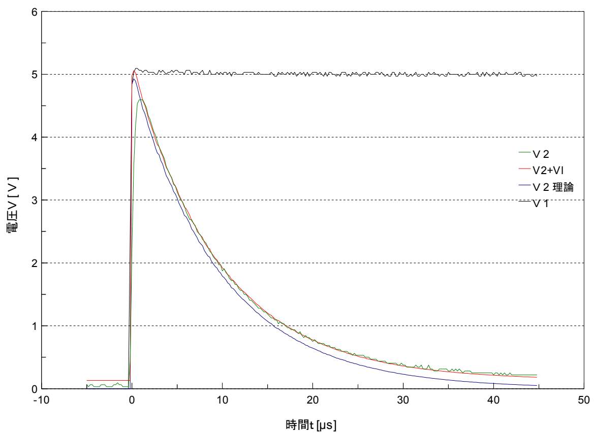
図7. 2 巻線抵抗による電圧効果を加味したRL回路の過渡応答
