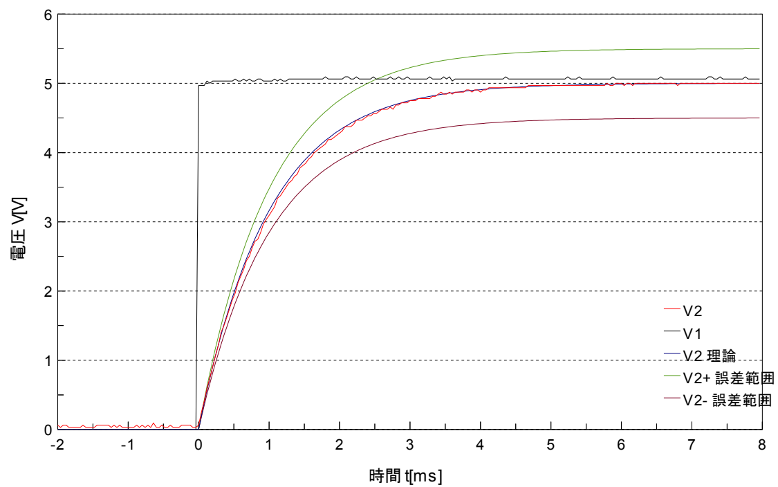
図7. 1 誤差範囲を考慮した RC 回路の過渡応答
