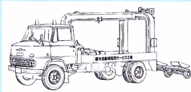
【LV-75a 日産C80型 3.5tトラック レッカー車(厚木自動車販売)】
