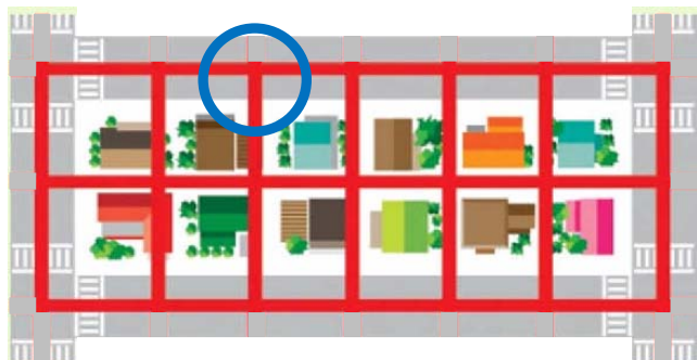
格子状地中壁工法の既存住宅地への適用イメージ※
